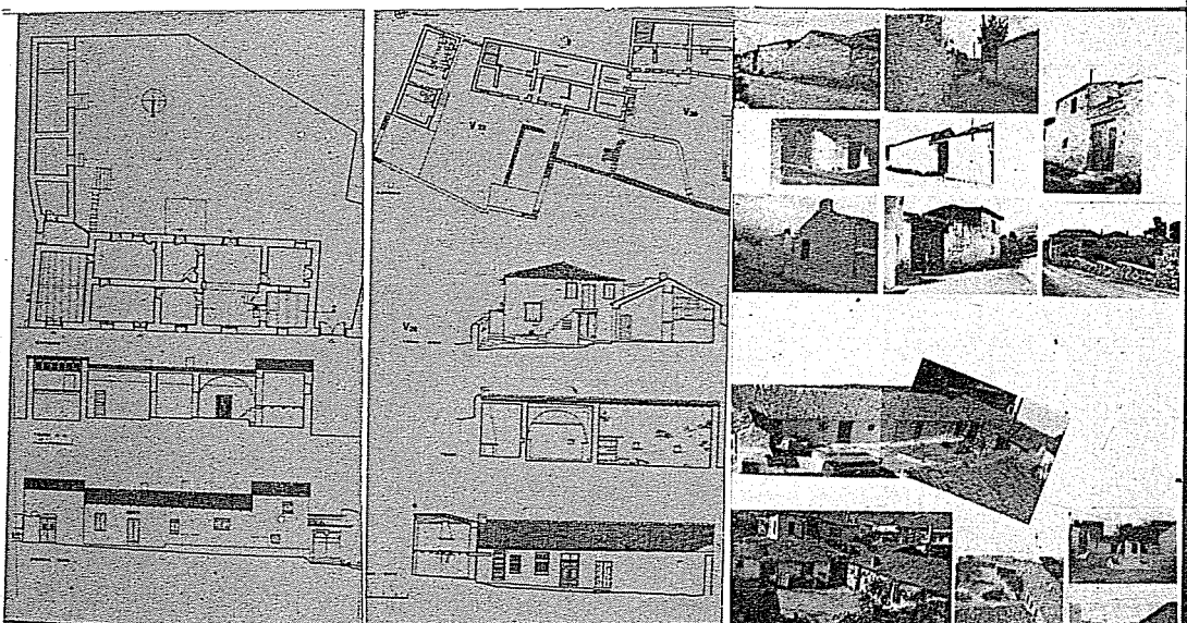
Εικ. 9. Σύνθετοι τύποι καμαρόσπιτου. Παραδείγματα, αριστερά στον Κουβαρά, δεξιά στην Παιανία.
