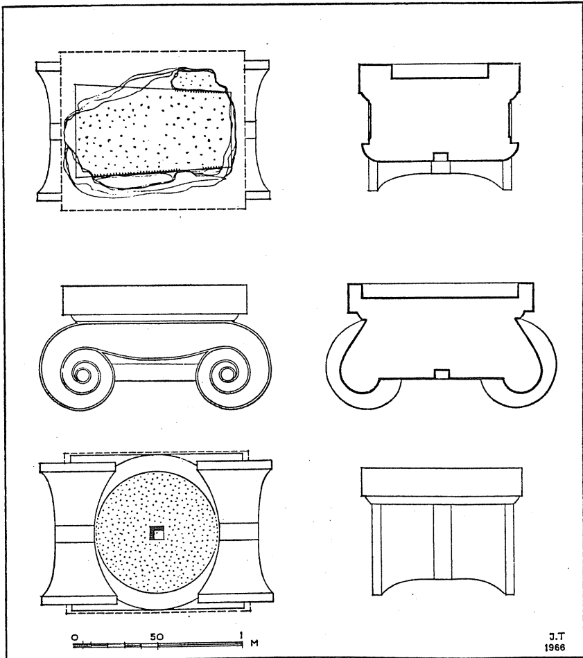
Εικ. 10: Ιωνικό κιονόκρανο, σχεδιασμένο από τον Ιω. Τραυλό (Vanderpool, Hesperia , 1966, p 98).
