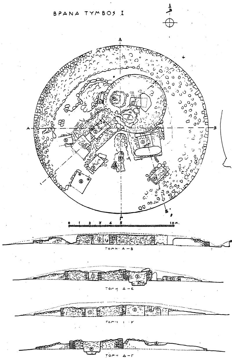
Εικ. 3: Βρανά, Τύμβος Ι. Κάτοψη και τομές (Μαρινάτος, ΠΑΕ 1970).
