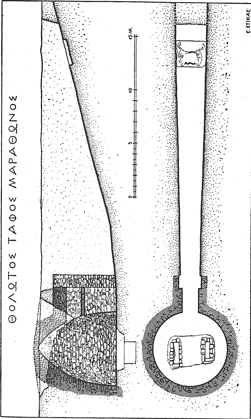
Εικ. 4: Οριζόντια και κατακόρυφη τομή του θολωτού τάφου του Μαραθώνα (ΠΙΛΕ 1958, σ. 17).
